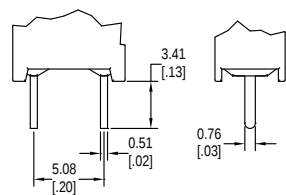
C SPST
