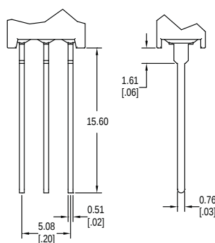
W SPDT
